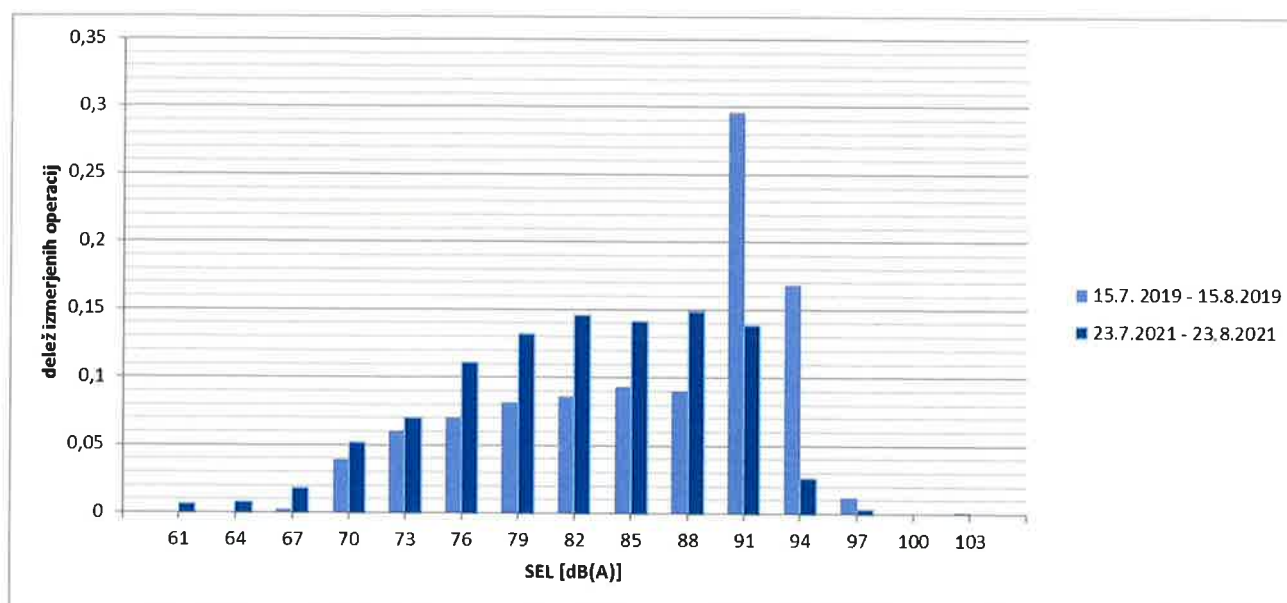
Slika 4.3: Porazdelitev ekspozicijskih ravni SEL letalskih operacij na merilnem mestu v Šenčurju za obdobje meritev med 23.7.2021 – 23.8.2021 ter 15.7.2019 – 15.8.2019.
