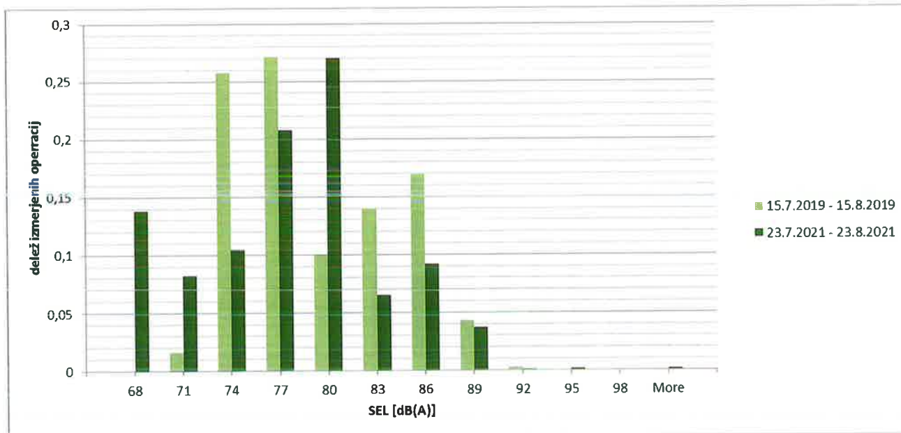
Slika 4.4: Porazdelitev ekspozicijskih ravni SEL letalskih operacij na merilnem mestu v Vodica - Lokarjih za obdobje meritev med 23.7.2021 – 23.8.2021 ter 15.7.2019 – 15.8.2019.
