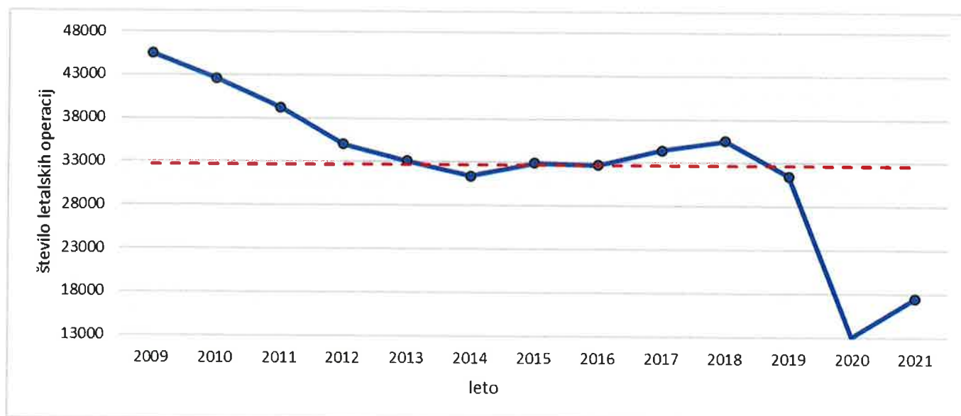
Slika 3.1: Število opravljenih letalskih operacij za obdobje 2009 – 2021.
