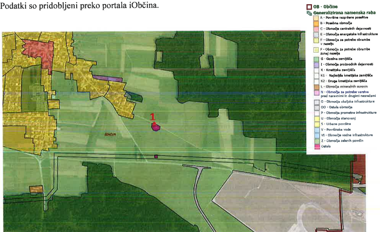
Slika 6.1: Območje merilnega mesta 1, v katerem se nahajajo objekti z varovanimi prostori, uvrščamo v območja III. stopnje varstva pred hrupom ( https://gis.iobcina.si , vir. 28.1.2021).
