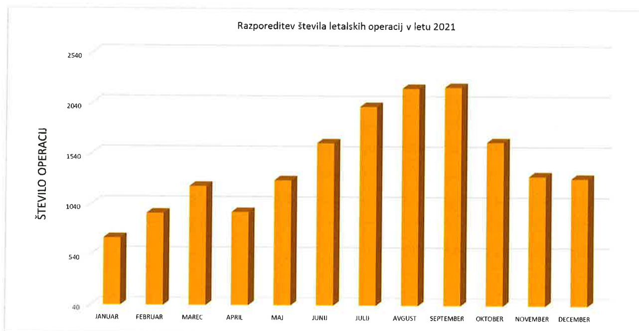
Slika 3.2: Razporeditev števila letalskih operacij tekom leta 2021.
