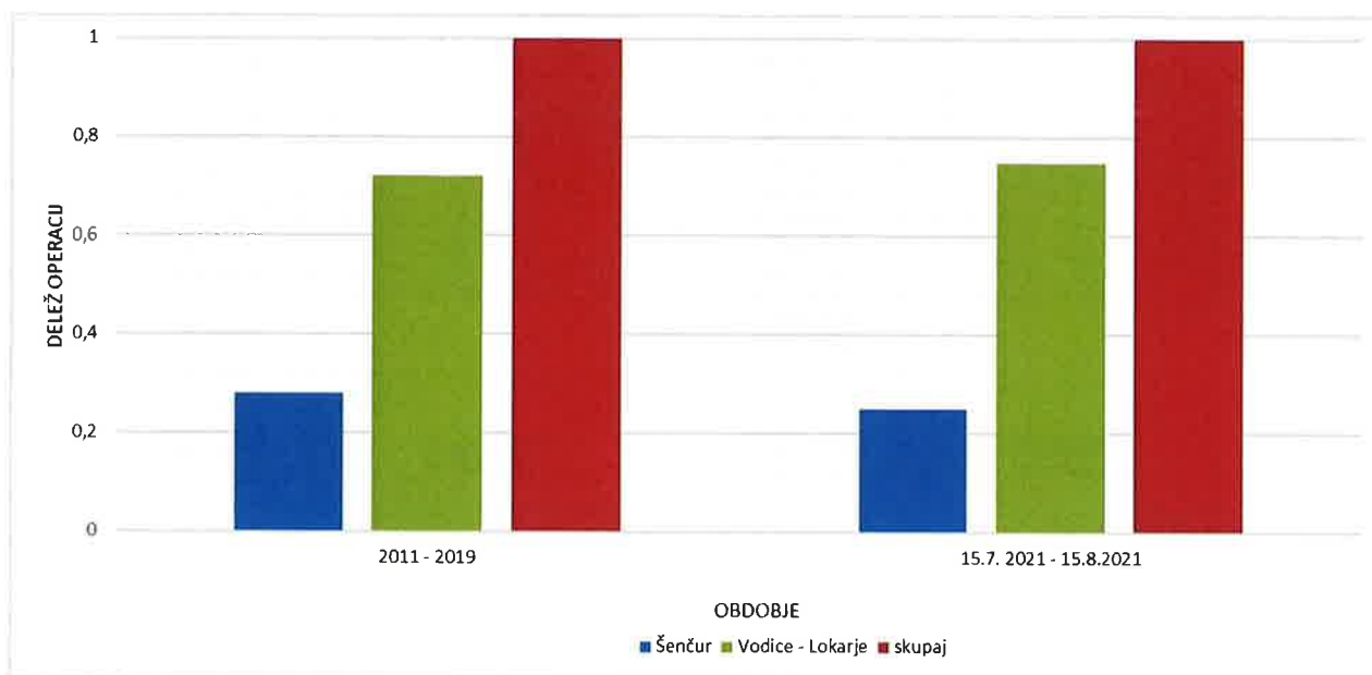
Slika 3.4: Deleži operacij v posamezni smeri za celotno obdobje meritev med 2011 - 2019 ter za obdobje 23.7.2021 – 23.8.2021.
