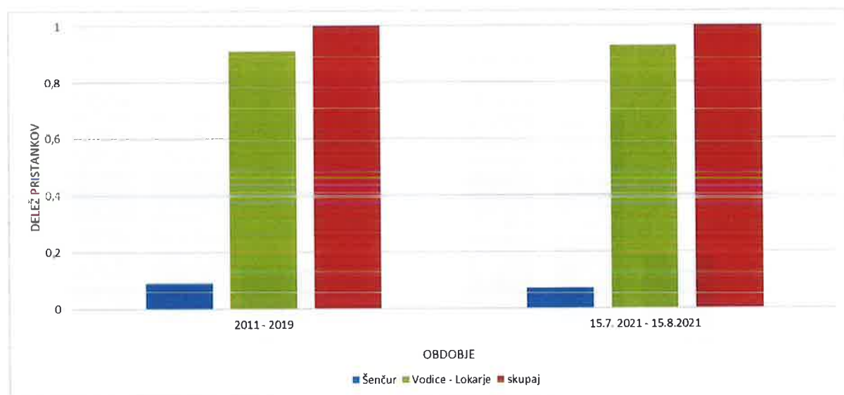
Slika 3.6: Deleži pristankov v posameznem obdobju za smer Šenčur in Vodice – Lokarje.
