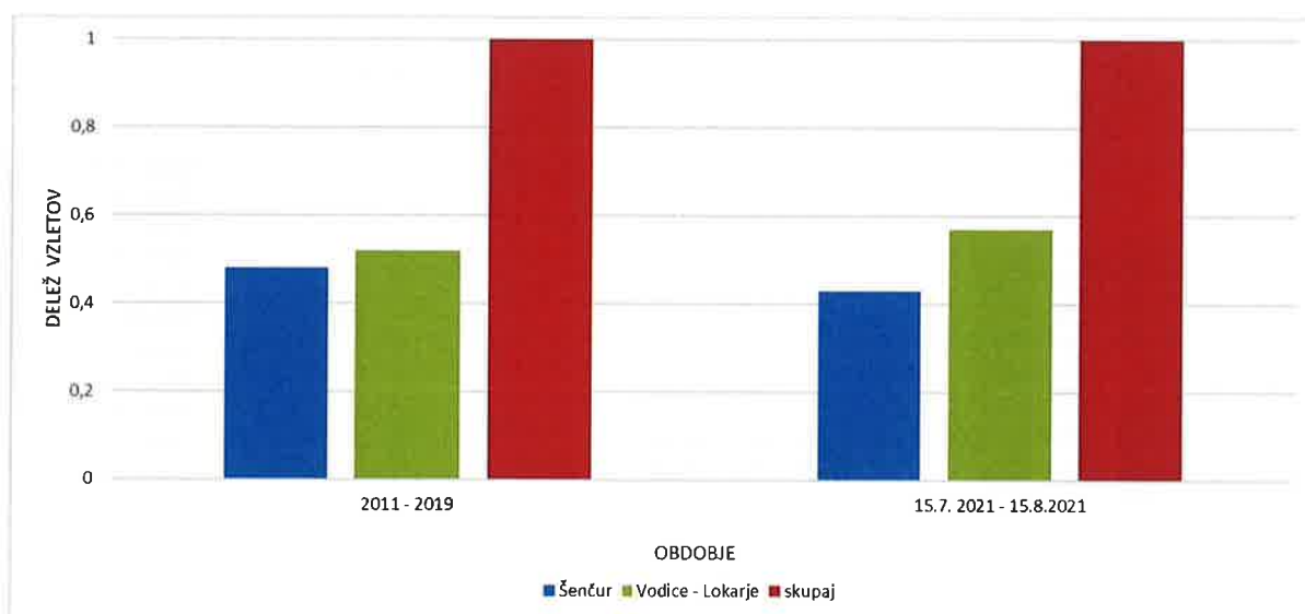
Slika 3.5: Deleži vzletov v posameznem obdobju za smer Šenčur in Vodice – Lokarje.
