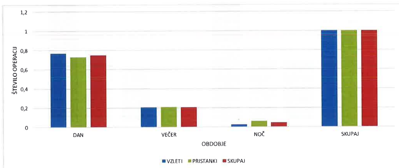
Slika 3.7: Deleži letalskih operacij, pristankov in vzletov v letu 2021 v posameznem obdobju dneva
