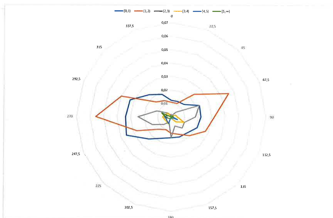
Slika 4.2: Roža vetrov za obdobje 23.7.2021 – 23.8.2021.
